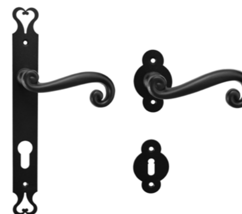
/// készleten SERRANO DDF hosszúcímes és díszes rozettás F fekete A fogantyú: zamak / cím: vas M A=105 mm B=250 mm C=30 mm D=50 mm
